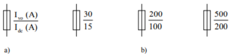
Hình 3-1. Ký hiệu đầy đủ cầu chì hạ áp và các ví dụ
