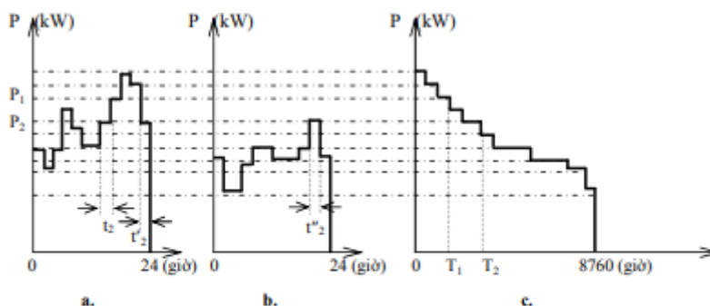
Hình 1-4: Đồ thị phụ tải hàng năm
