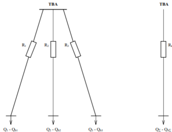
Hình 4-11. Sơ đồ thay thế và sơ đồ tương đương lưới điện hạ áp dùng xác định Q_{bi}
