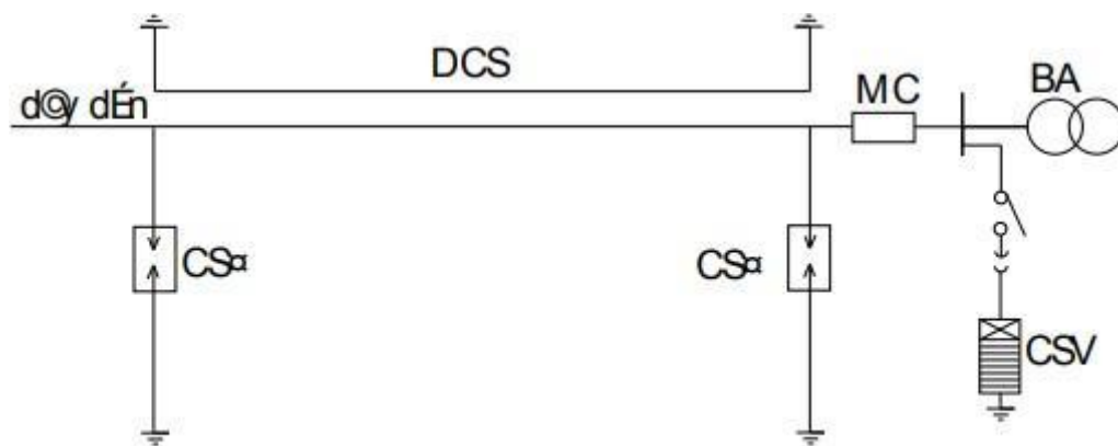
Hình 3-14. Sơ đồ bảo vệ trạm 35 ÷ 110kV
