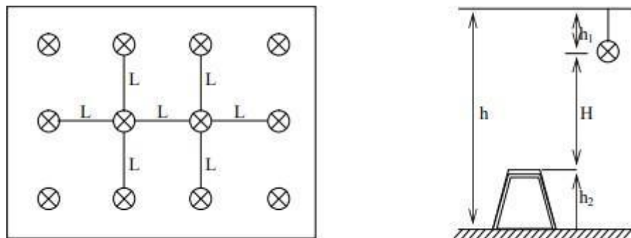
Hình 4-4. Bố trí đèn trên mặt bằng và mặt đứng
