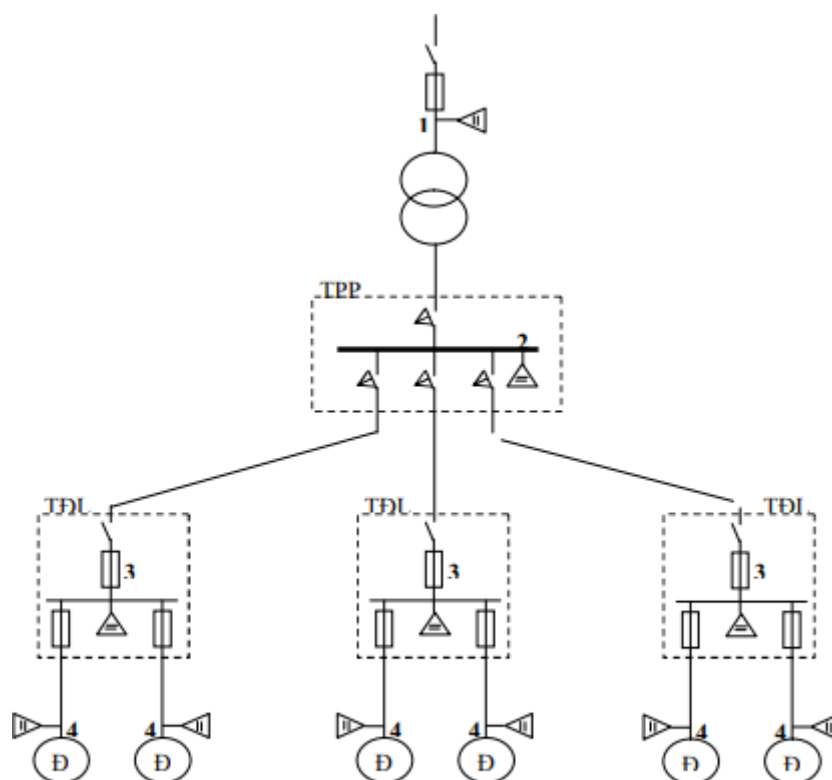
Hình 4-9. vị trí đặt tụ bù trên lưới điện xí nghiệp
