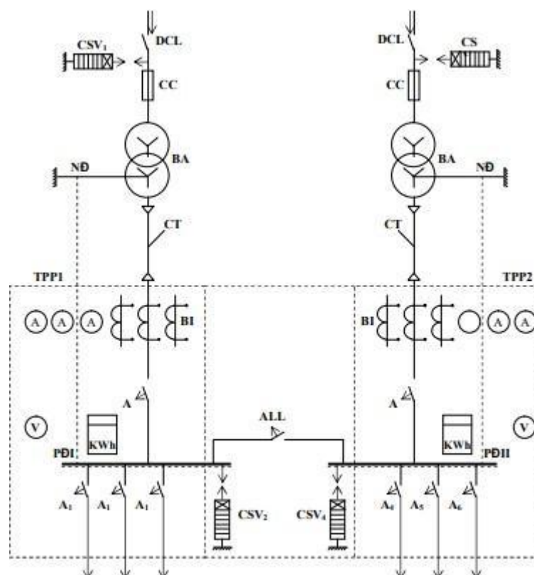
Hình 2-15. Sơ đồ nguyên lý trạm biến áp phân phối hai máy
