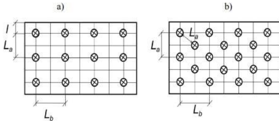
Hình 4-1. Cách bố trí đèn: a) Theo hình chữ nhật, b) Theo hình thoi.
