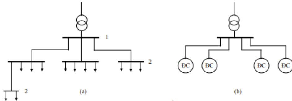
Hình 1-9. Sơ đồ hình tia a. Cung cấp điện cho phụ tải phân tán b. Cung cấp điện cho phụ tải tập trung 1. Thanh cái trạm biến áp phân xưởng. 2. Thanh cái tủ phân phối động lực
