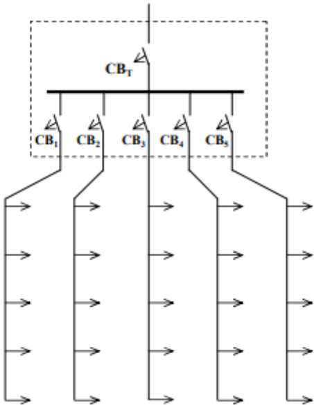
Hình 4-3. Sơ đồ nguyên lý cấp điện chiếu sáng cho siêu thị
