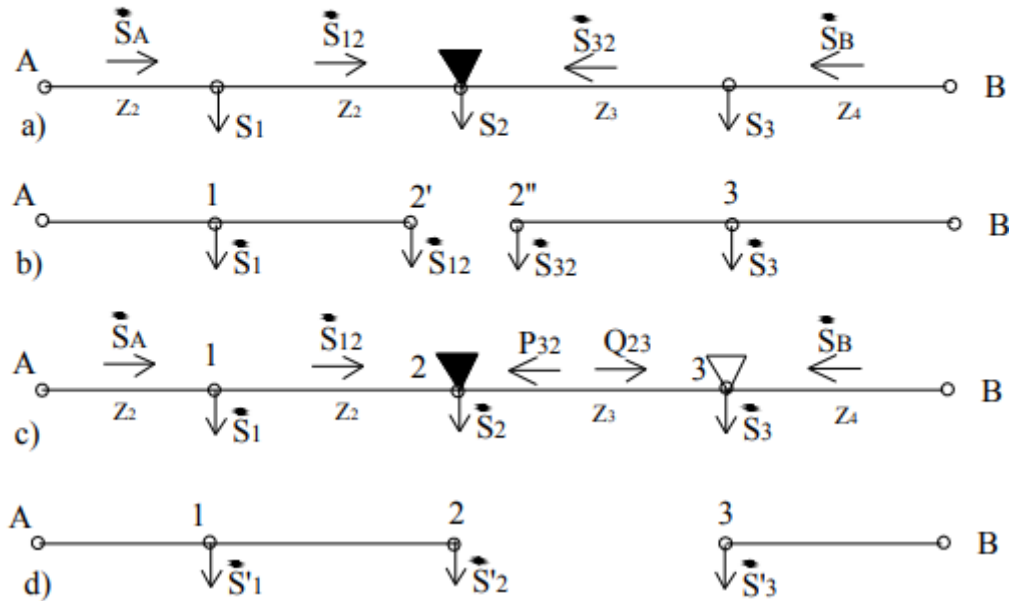
Hình MĐ 19-03-08: Các điểm phân bố công suất tác dụng và công suất phản kháng
