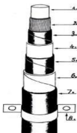
Hình 3-22. Dây dẫn đưa dòng điện sét xuống đất gồm nhiều lớp, trong đó có phần dẫn chính là vành đồng tiết diện 50mm 2 và có màn chắn bằng băng đồng.
