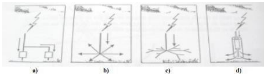
Hình 3-26a. Một phương pháp có hiệu quả của cọc nối đất – dòng điện đi xuống đất được rẽ nhánh.
