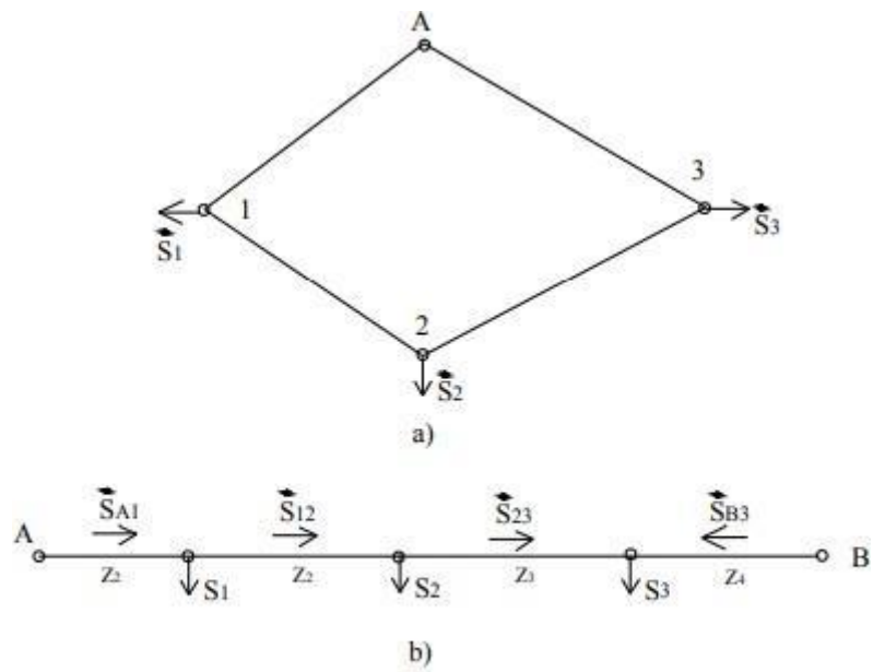
Hình 2-7. Mạng kín có ba phụ tải
