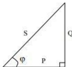
Hình 4-7. Tam giác công suất
