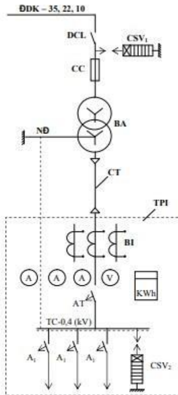
Hình 2-14. Sơ đồ nguyên lý trạm biến áp phân phối một máy
