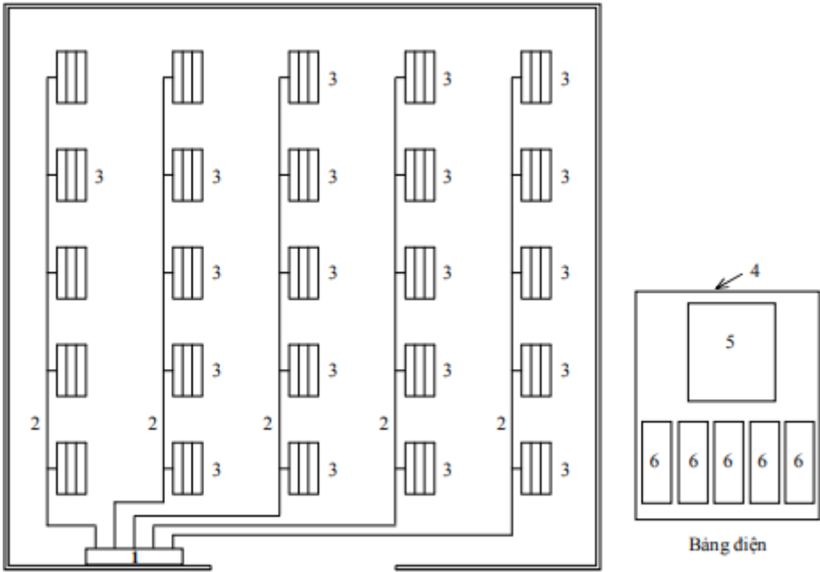
Hình 4-2. Sơ đồ mặt bằng bố trí đèn và đi dây
