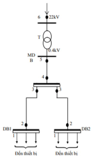
Hình 1-6. Sơ đồ nguyên lý cung cấp điện
