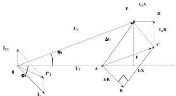
Hình 2-1. Véc tơ tổn thất điện áp
