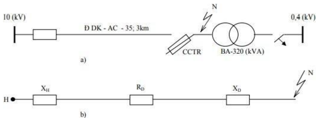
Hình MD 19-04-03: Sơ đồ nguyên lý và sơ đồ thay thế tính ngắn mạch
