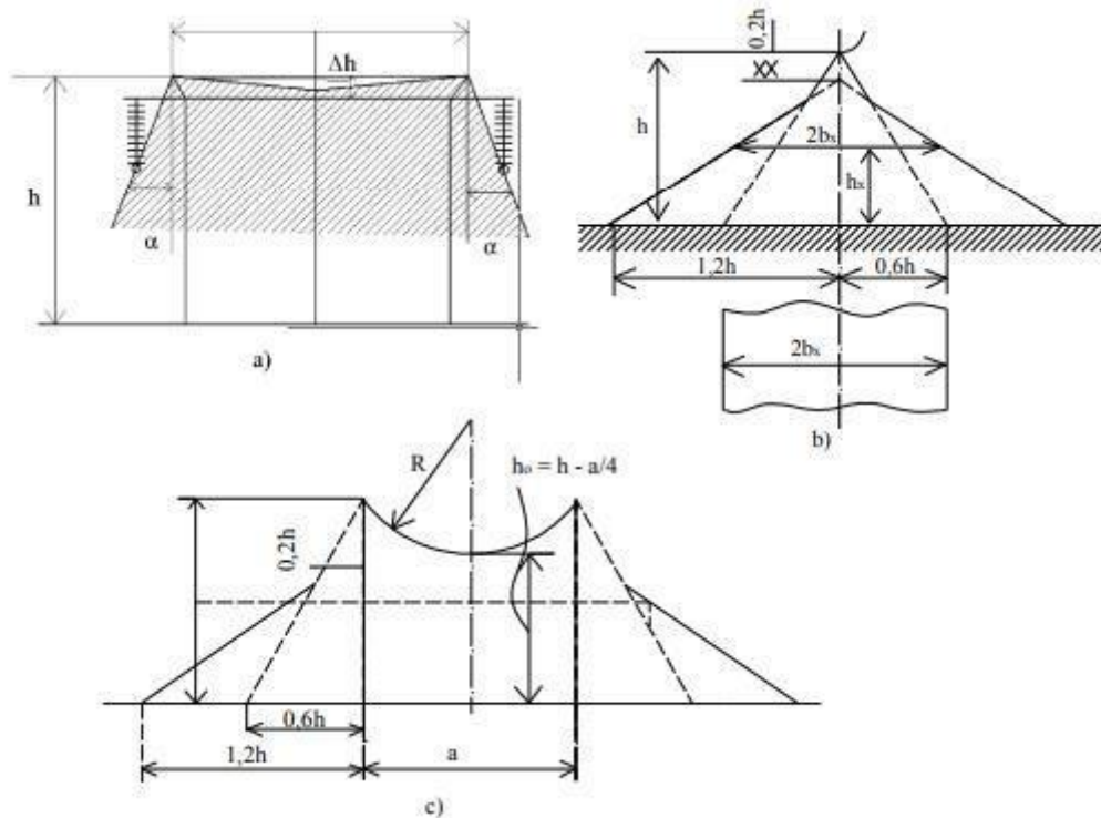
Hình 3-10. Góc bảo vệ và phạm vi bảo vệ của dây chống sét
