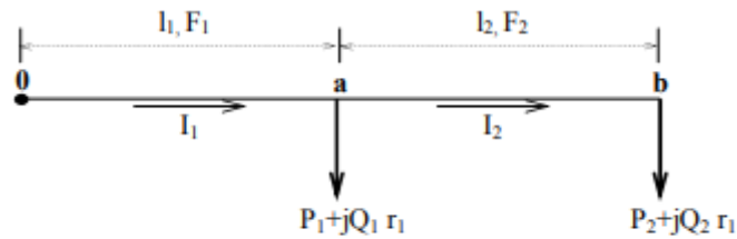
Hình 3-8. Sơ đồ mạng cung cấp điện
