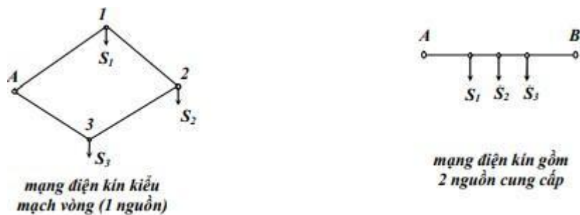
Hình 2-5. Sơ đồ mạng điện kín
