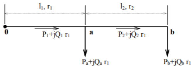
Hình 3-6. Sơ đồ mạng cung cấp điện
