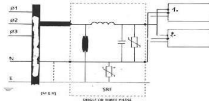
Hình 3-29. Sơ đồ nguyên lý bộ lọc làm giảm sự tăng cao SRF (Surge Reduction Filters) dùng để bảo vệ các đường dây điện lực đi đến.
