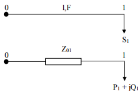
Hình 2-2. Sơ đồ nguyên lý và sơ đồ thay thế đường dây 1
