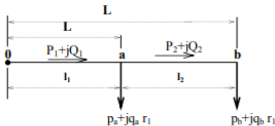
Hình 3-7. Sơ đồ cung cấp điện
