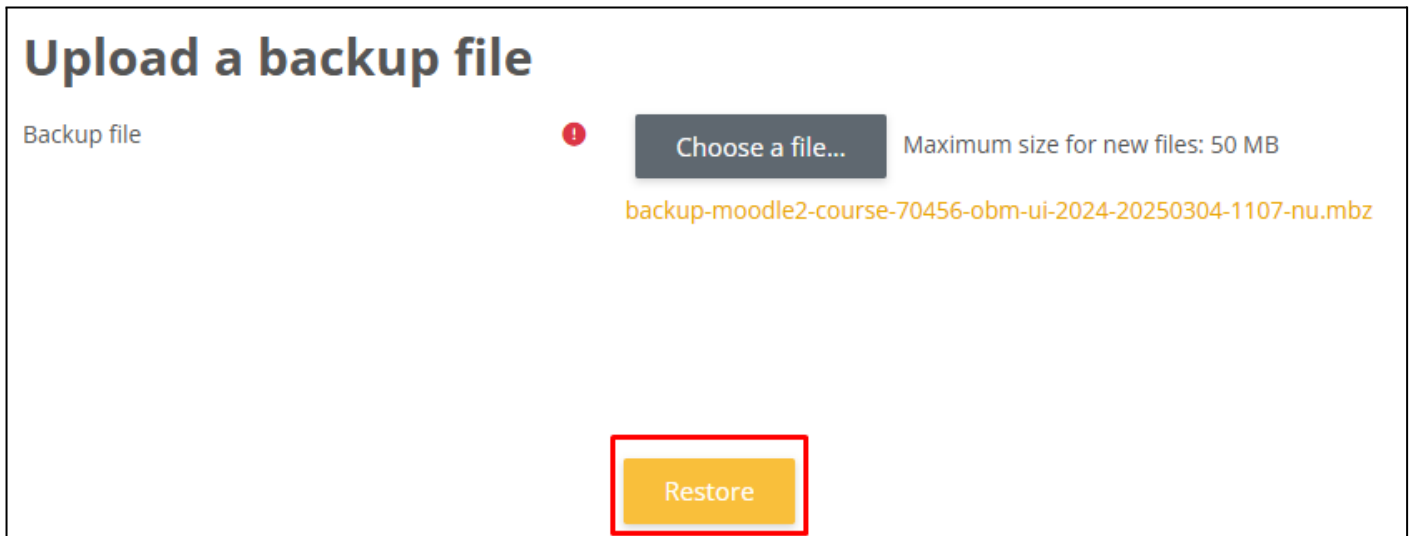
Gambar 14. Restore
