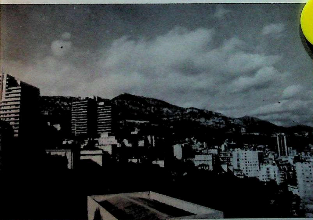
Monte Carlo
