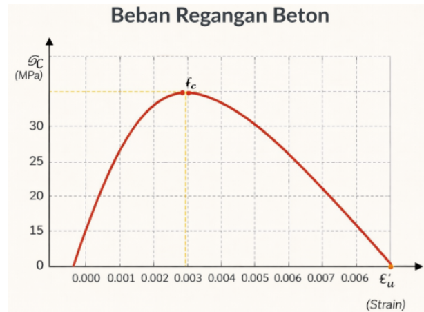
Gambar 2 Beban Regangan Beton
