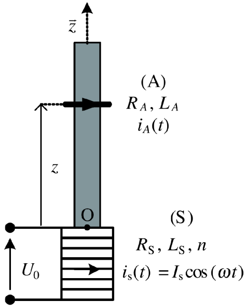
Figure 2 : Une réalisation de l'expérience d'Élihu Thomson.
