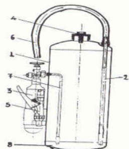
Πυροσβεστήρας ξηράς σκόνης με εξωτερικό φιαλίδιο CO 2
