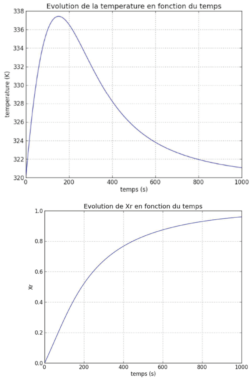
Figure 5 – Température et conversion calculées à partir du modèle constitué du système d'équations différentielles déterminées dans la Partie I
