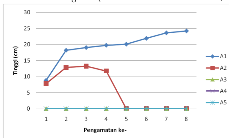
Gambar 1. Pengaruh pemberian abu terhadap tinggi bibit kakao
