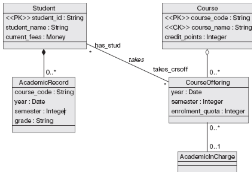
Рис. 10. Специфікація агрегацій (Запис на університетські курси)
