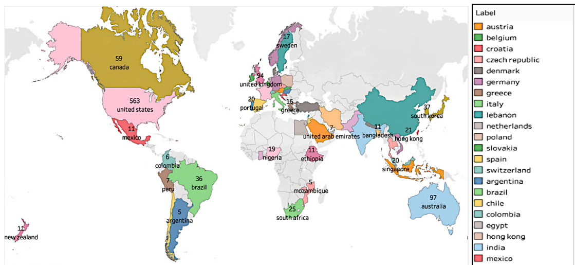
Gambar 1. Kontibusi dari berbagai Negara terkait Penelitian Hipertensi
