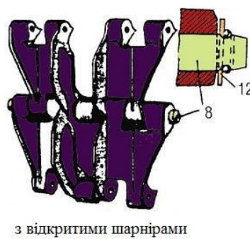
ТИПИ ГУСЕНИЦЬ
