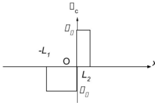
Figure 2 : profil de densité de charges dans la jonction PN
