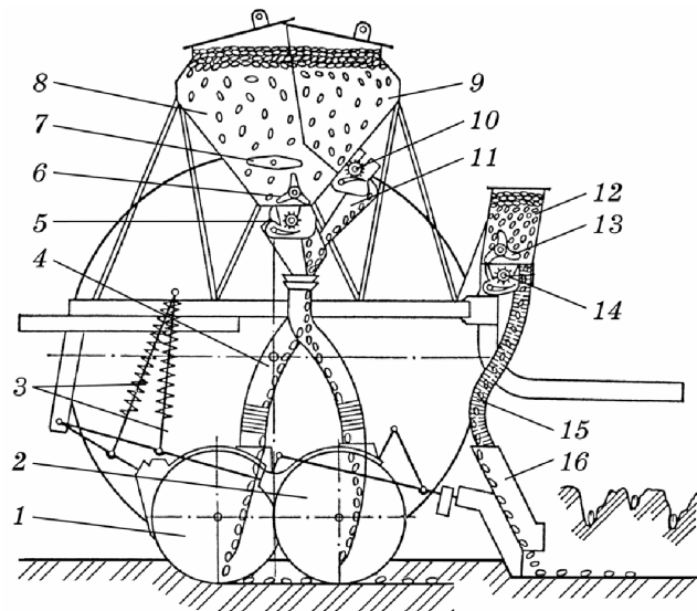
Рис. 3.7. Функціональна схема зернотукоп'яної сівалки СЗТ-3,6А: 1 і 2 — дискові сошники; 3 — штанги з пружинами; 4 і 15 — насіннепроводи; 5 і 14 — насінневисівні апарати; 6 і 13 — нагнітачі; 7 — ворушилка; 8 і 9 — відділення ящика зернотукоп'яного і для добрив; 10 — туковисівний апарат; 11 — лотік; 12 — ящик для насіння трав; 16 — кілеподібний сошник
