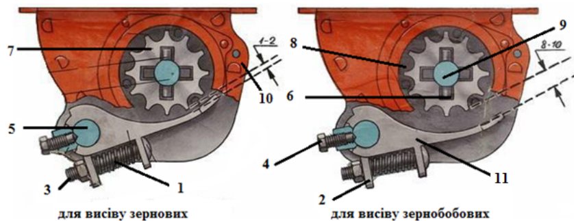
Рис. 3.3. Котушковий висівний апарат сіялки СЗ-3,6А:
