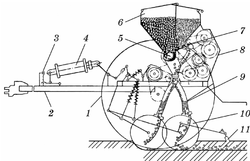
Рис. 3.2. Зернотукова сівалка СЗ-3,6А:
