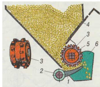
Рис. 3.4. Котушковий туковисівний апарат сіялки СЗ-3,6А:
