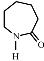
caprolactam (vòng) ;
