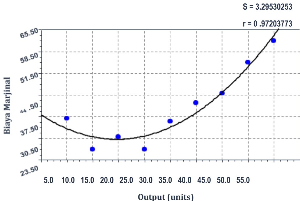
Gambar 1. Kurva Biaya Marjinal dan Output suatu proses produksi
