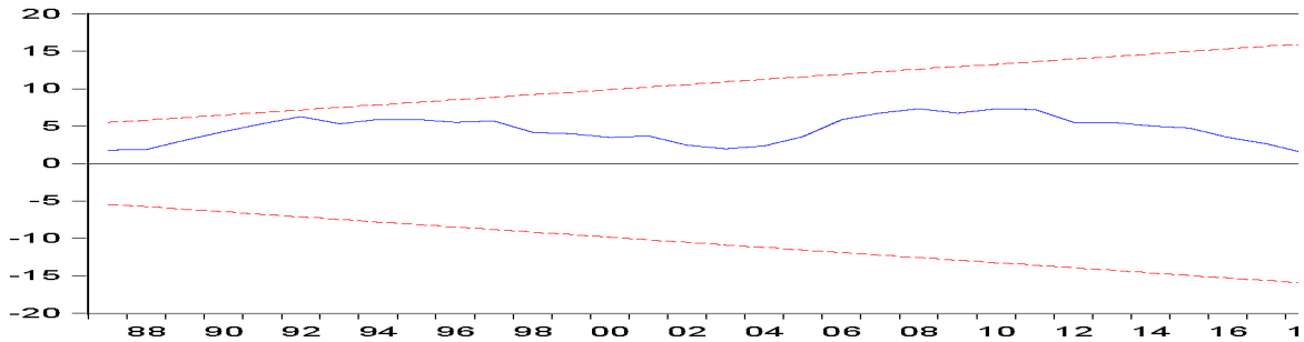
Grafik 1: Cusum Grafiği
