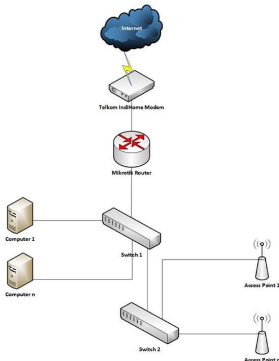
Gambar 1. Skema dari Topologi Jaringan yang diteliti
