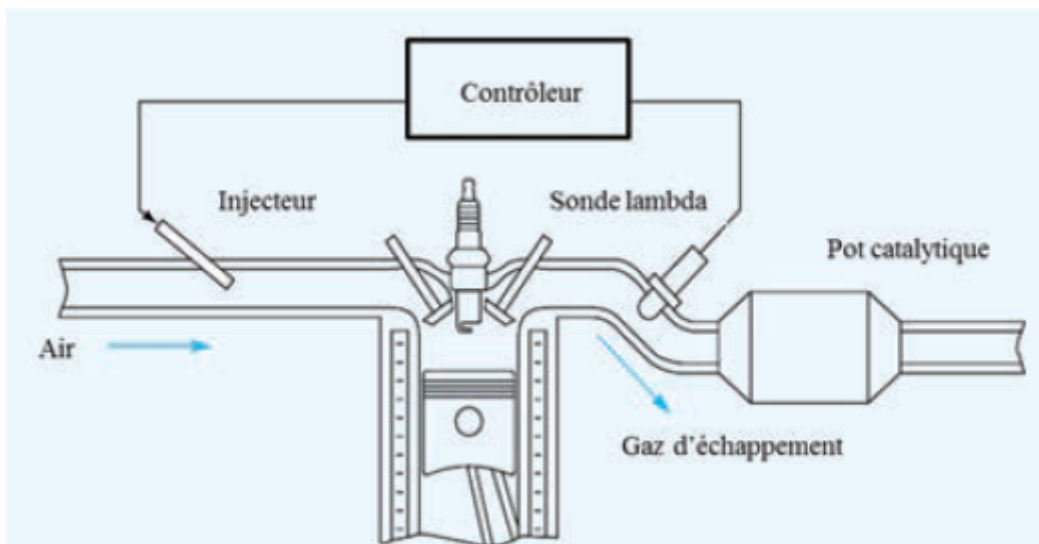
figure 4 : principe du contrôle en boucle fermée.
