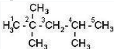
2,2,4-триметилпентан
