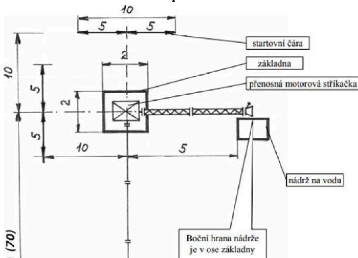
obr. 1 plán trati
