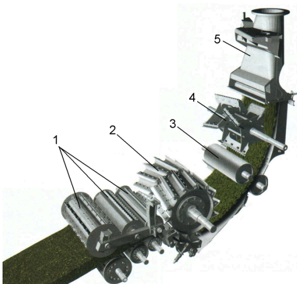
Рис.20. Подрібнюючий апарат кормозбирального комбайна BIG X (KRONE):
