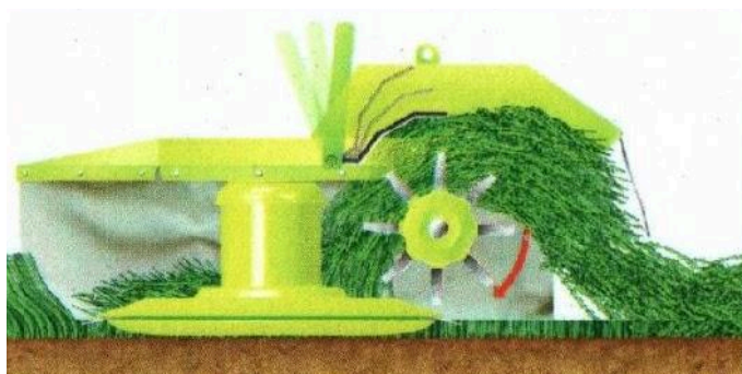
Рис. 6. Робота барабанної косарки в агрегаті з плющилкою.
