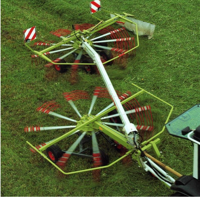
Рис. 8. Двороторні граблі LINER 650 TWIN CLAAS (Німеччина).
