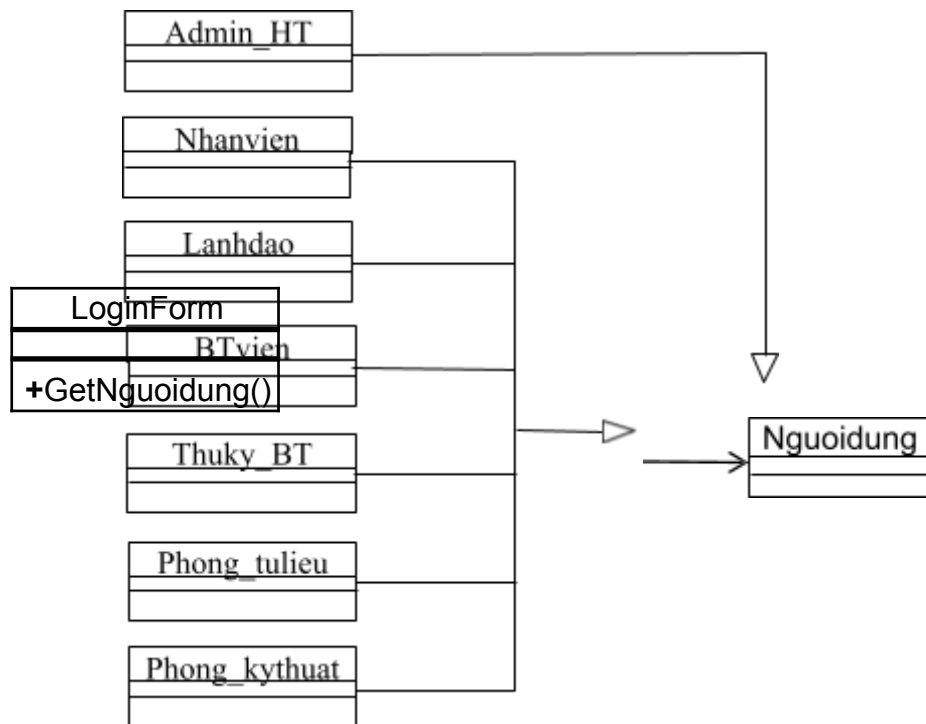
Hình 3.12: Áp dụng mẫu Factory trong pha login
