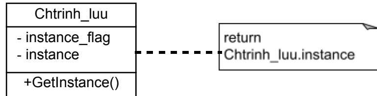
Hình 3.13: Khi áp dụng mẫu đơn chiếc cho lớp Chtrinh_luu.
