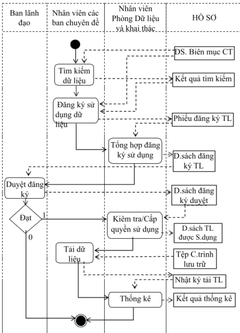
Hình 3.3: Sơ đồ tiến trình nghiệp vụ “Quản lý sử dụng dữ liệu”
