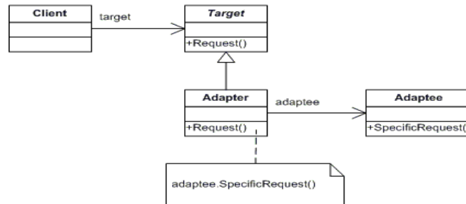
Hình 2.7: Biểu đồ lớp thích nghi
