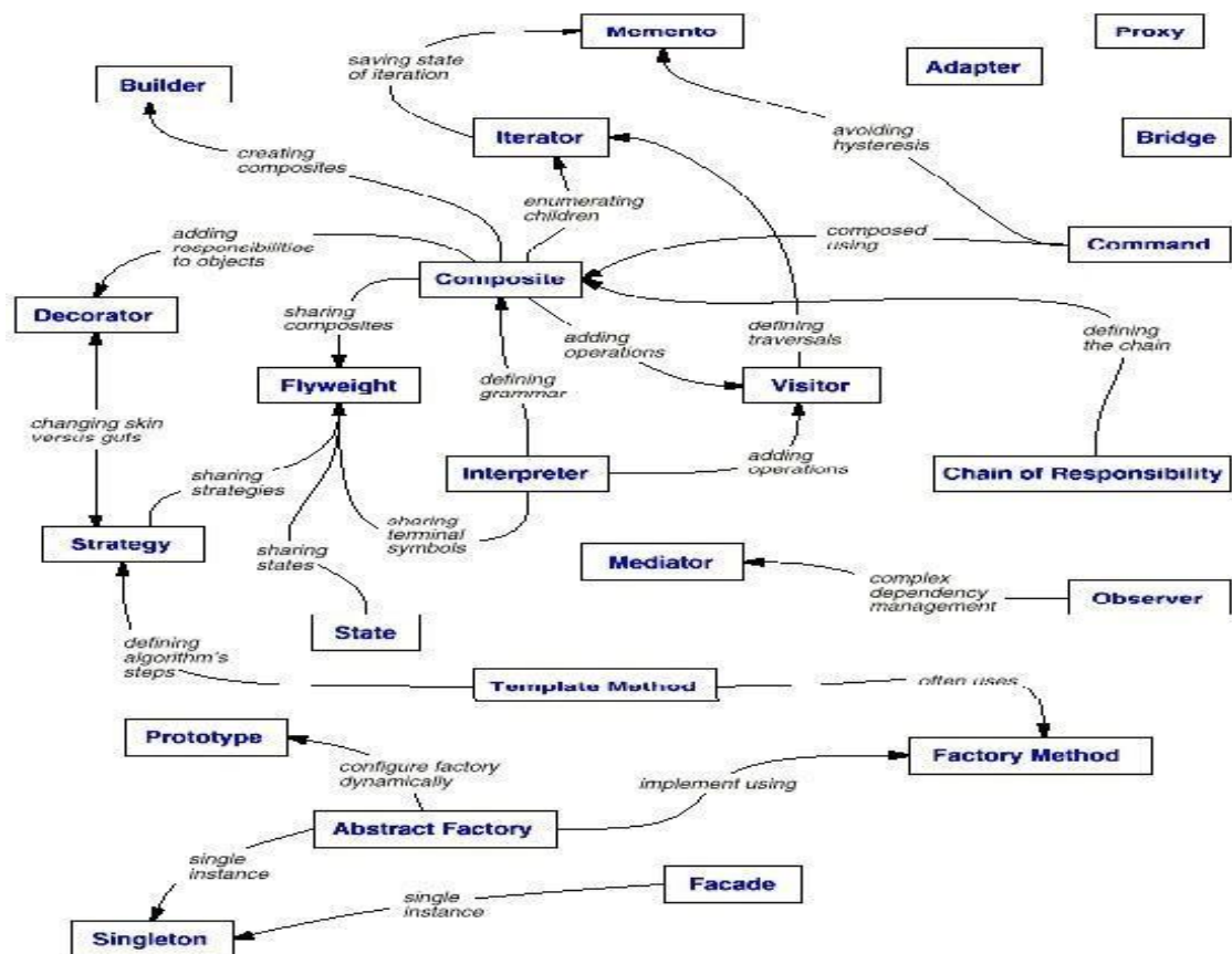
Hình 2.8: Sơ đồ mối liên kết các mẫu thiết kế
