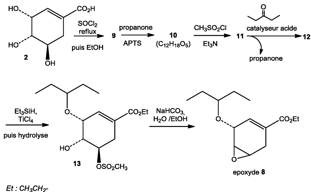
Schéma 7 : voie de synthèse de l'époxyde 8
