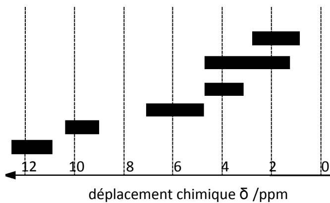
Figure 1 : Plages de déplacements chimiques en spectroscopie de RMN du proton pour certains groupes de protons caractéristiques (référence tétraméthylsilane : \delta = 0 ppm ; X=hétéroatome)
