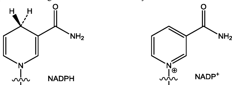
Schéma 4 : structures de NADPH et NADP +
