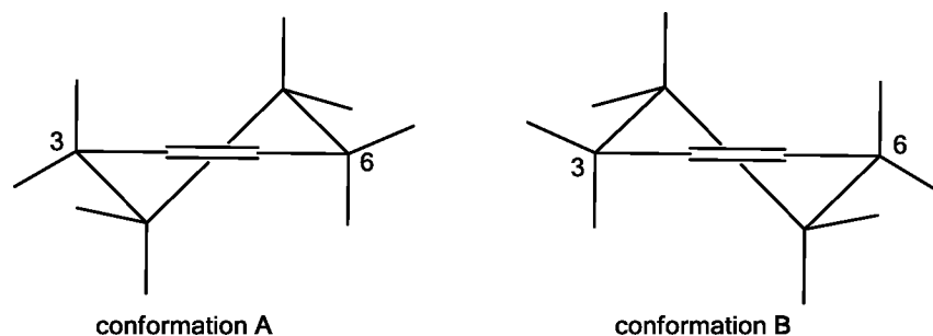
Schéma 5 : conformations stables de 2
