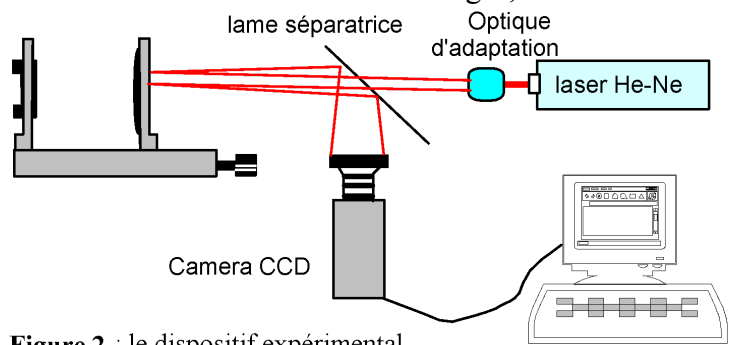
Figure 2 : le dispositif expérimental
