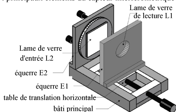
Figure 1 : principaux éléments du capteur interférométrique
