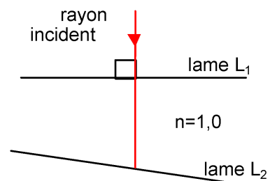
Figure 10: interféromètre réglé en coin d'air
