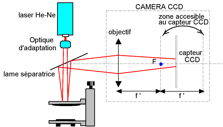
Figure 7 : enregistrement de la figure d'interférence
