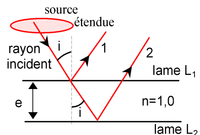
Figure 6 : lame d'air et source étendue à distance finie
