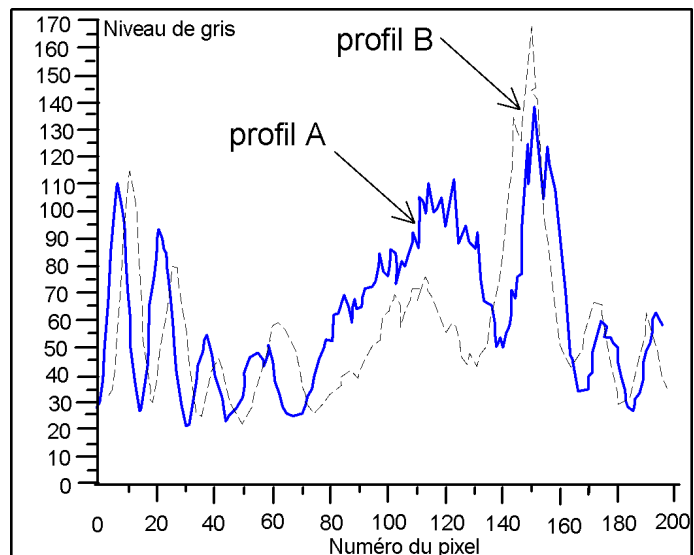
Figure 8 : enregistrement du déplacement des franges circulaires
