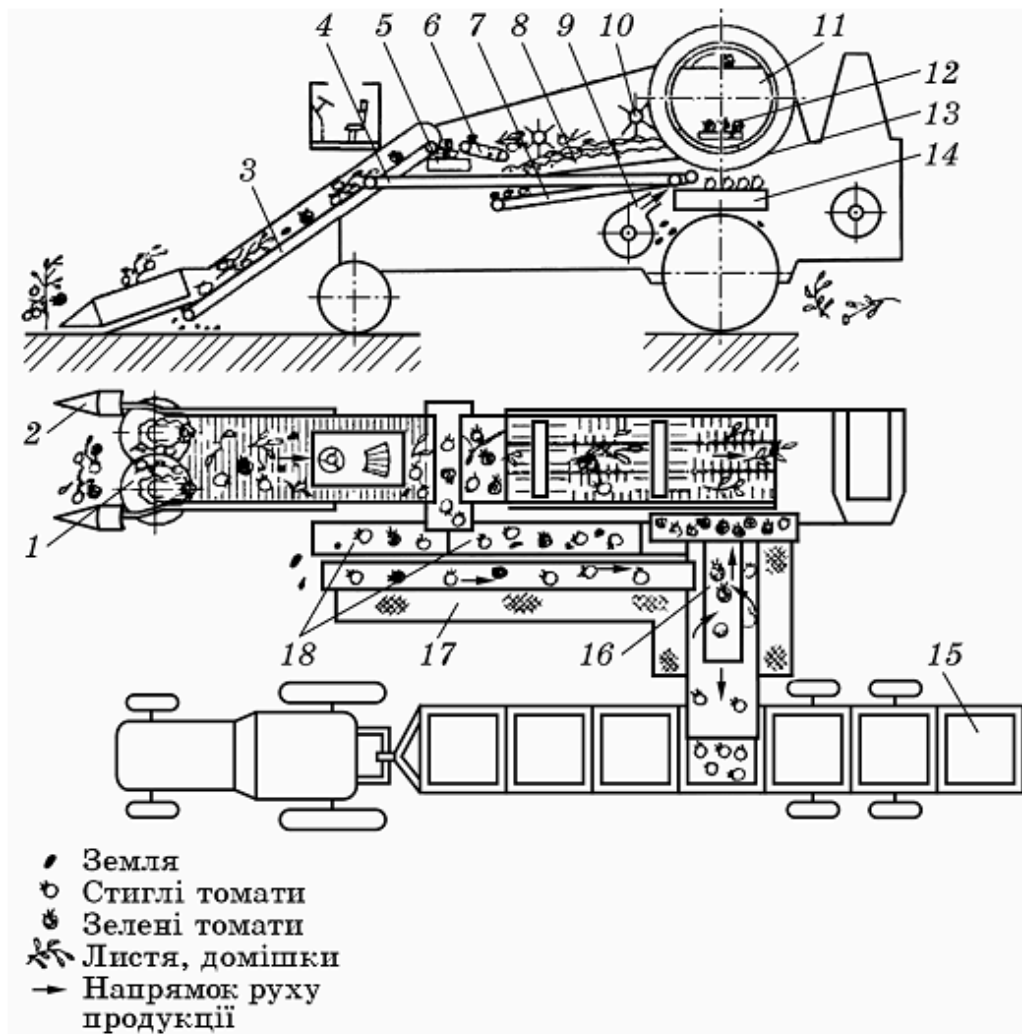
Рис.1. Схема тоmatозбирального комбайна СКТ-2:
