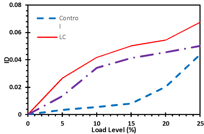
Gambar 2. ID ( index of damage ) dari data acoustic emission (AE) (nama tahun)
