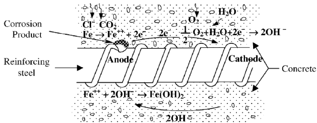
Gambar 1. Proses korosi pada beton (nama, tahun)
