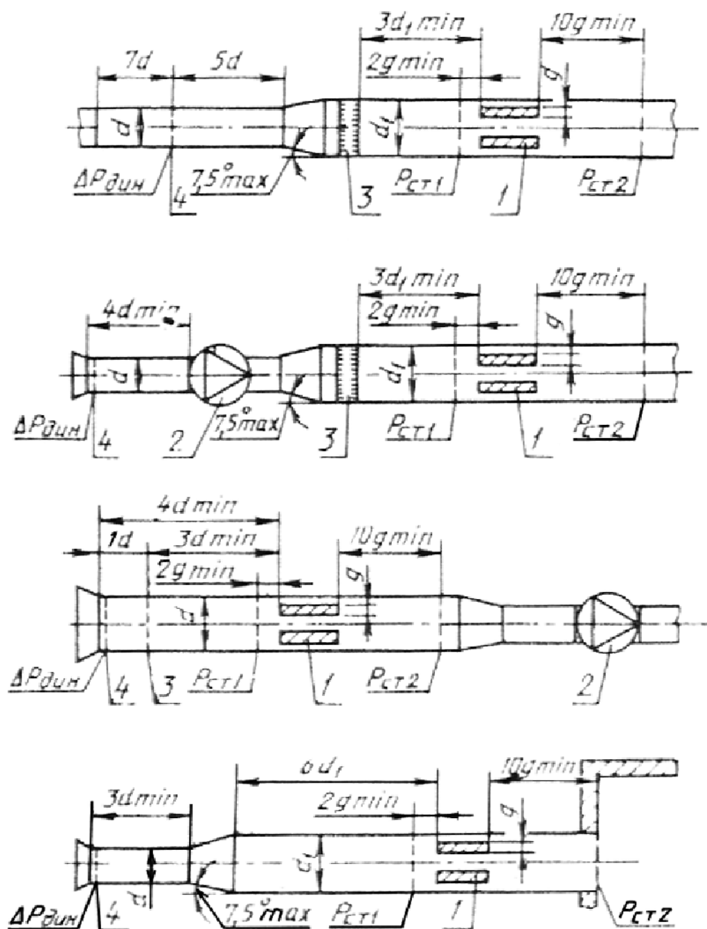
1 - испытываемый глушитель шума; 2 - вентилятор; 3 - направляющая решетка; 4 - измерительное сужающее устройство или сопло
