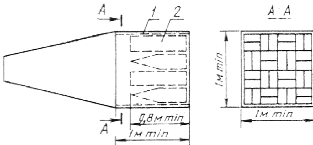
1 - звукопоглощающий материал; 2 - поглощающий клин Черт. 3
