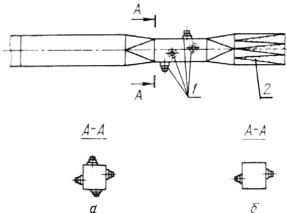
Примеры решений измерительных источников звука
