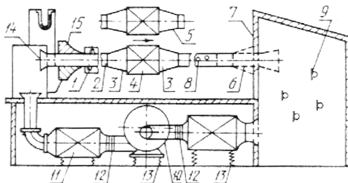
Испытательный стенд для измерения уровней звуковой мощности собственного шума глушителя
