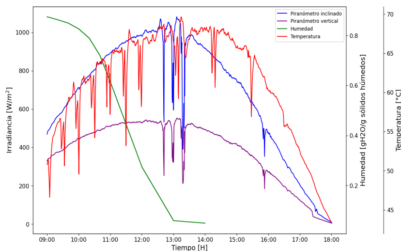
Figura 1. Cinética de secado de cempasúchil ( Tagetes erecta L.) realizada en un secador solar de modo mixto el día 21 de octubre de 2024.
