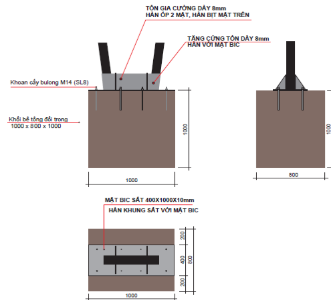
CT-ĐẾ ĐÓ BÊ TON ẨM MẶT BẰNG ĐẤT KHOAN CÂY BULÔNG M14
