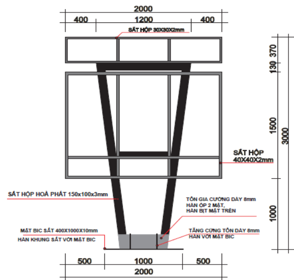
MẶT ĐỪNG KẾT CẤU KHUNG SẮT
