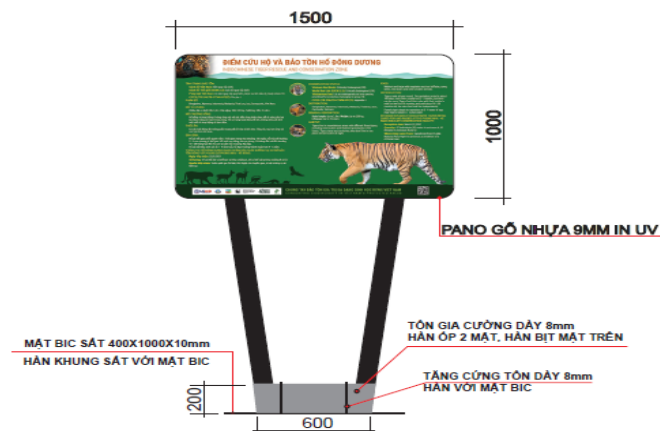
MẶT ĐỨNG DEMO BIÊN
