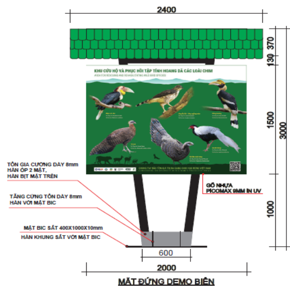
MẶT ĐỪNG DEMO BIÊN
