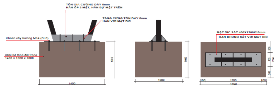
CT-ĐẾ ĐÓNG BÊTÔNG ẨM MẶT BẰNG ĐẤT KHOAN CÂY BULÔNG M14
