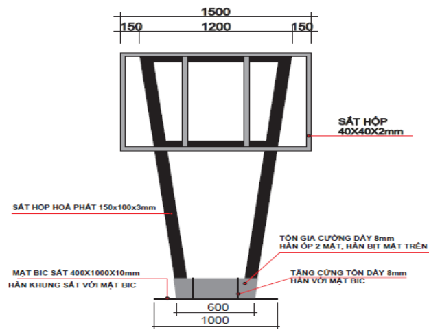
MẶT ĐỪNG KẾT CẤU KHUNG SẮT
