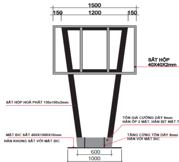
MẶT ĐỨNG KẾT CẤU KHUNG SẮT
