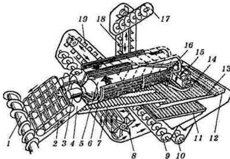
11 Схема молотарки комбайна TR-70:
