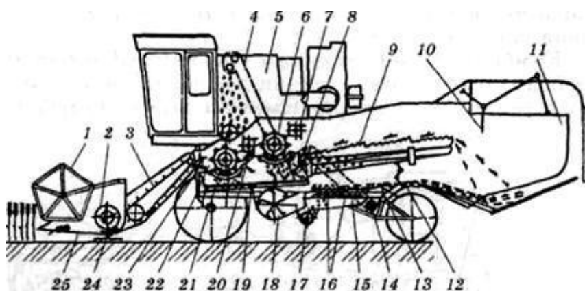
3 Технологічна схема комбайна «Енисей-1200»:
