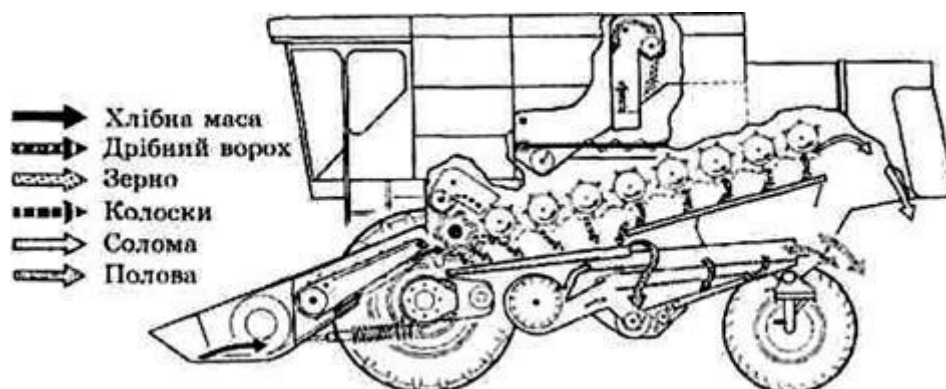
8 Схема технологічного процесу комбайна «Командор 228»
