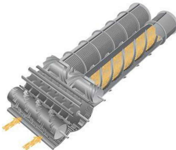
9 Молотильно-сепарувальний пристрій Комбайна LEXION 480
