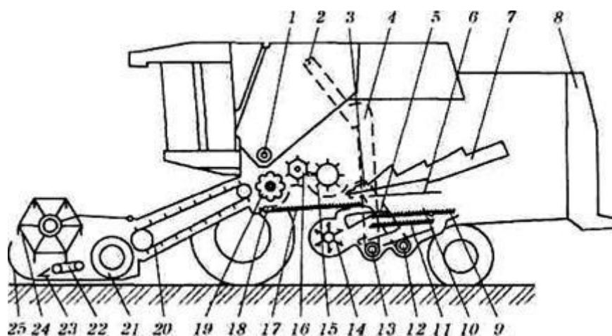
7 Технологічна схема комбайна «MF-36» фірми «Массей Фергюсон»:
