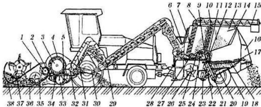
14 Схема технологічного процесу роботи зернозбирального комплексу КЗС-10:
