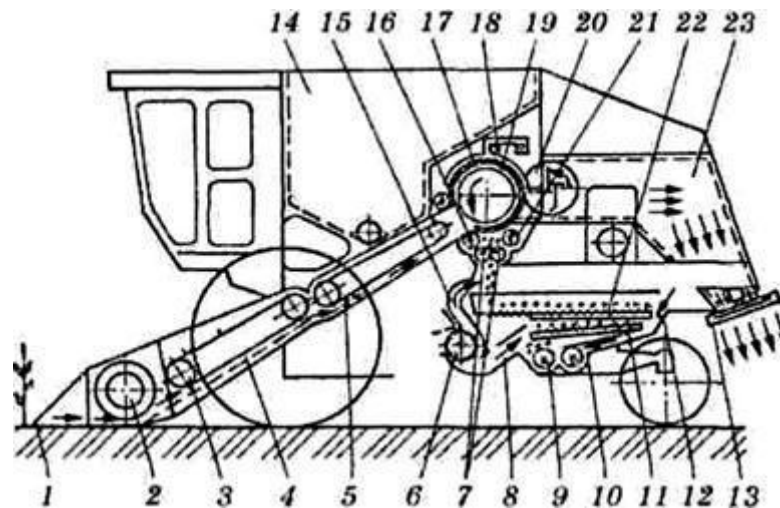
12 Технологічна схема комбайна «Allis Chalmers» № 6:
