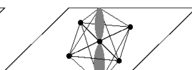
AX_4E_2 carré
