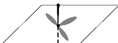
AX_2E_3 linéaire
