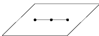
AX_2E_0 linéaire
