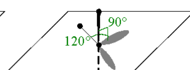
AX_3E_2 en T
