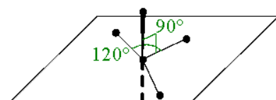
AX_5E_0 bipyramide trigonale
