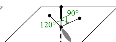
AX_4E_1 tétraèdre non régulier
