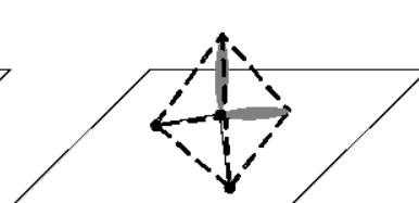
AX_2E_2 coudée
