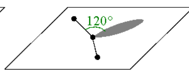
AX_2E_1 coudée
