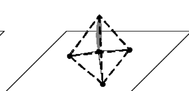
AX_5E_0 pyramide à base triangulaire
