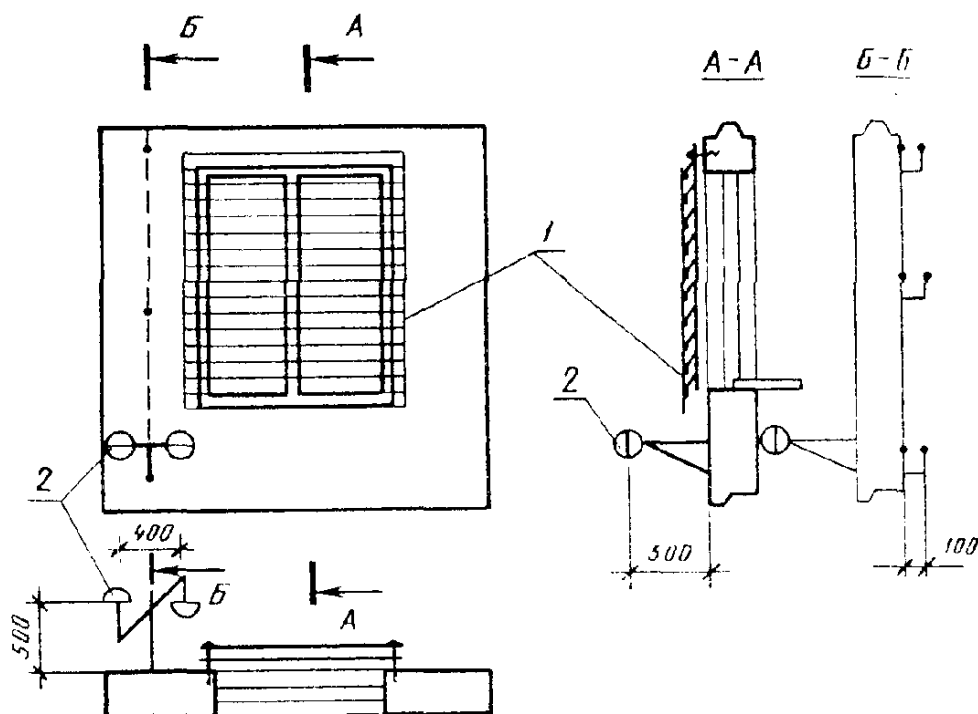
Схема установки пиранометров
