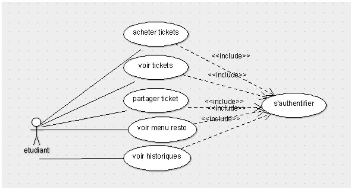
Fig 1: Diagramme des cas d'utilisations pour étudiant
