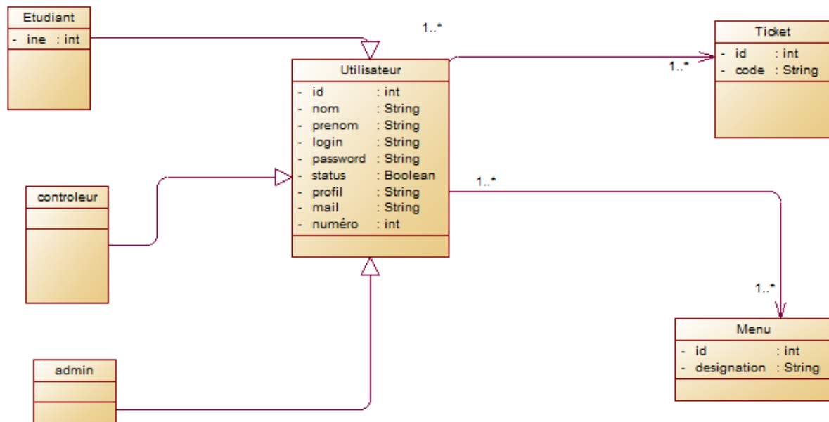
Fig 3 : Diagramme de classe
