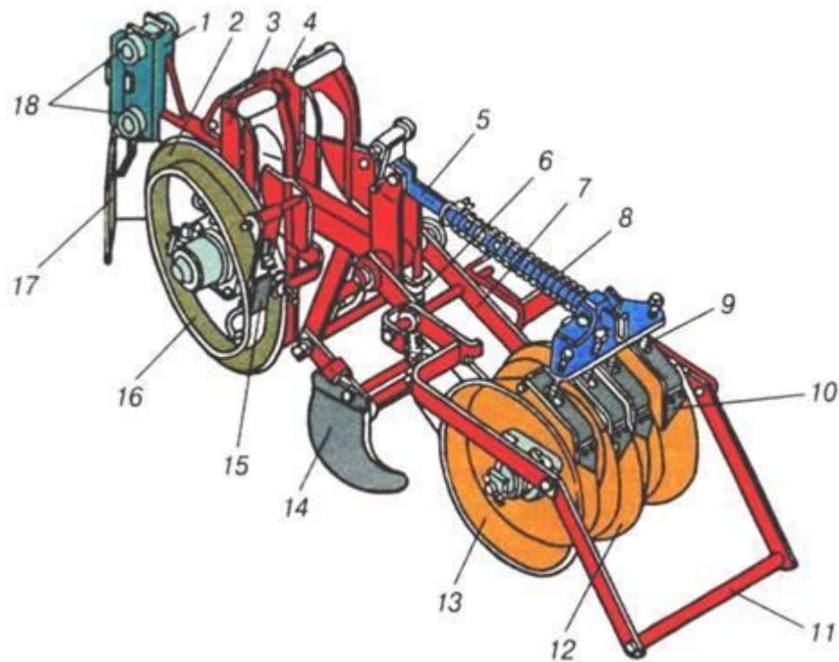
Рис. 7. Дворядковий дисковий сошник сівалки СОН-4,2:
