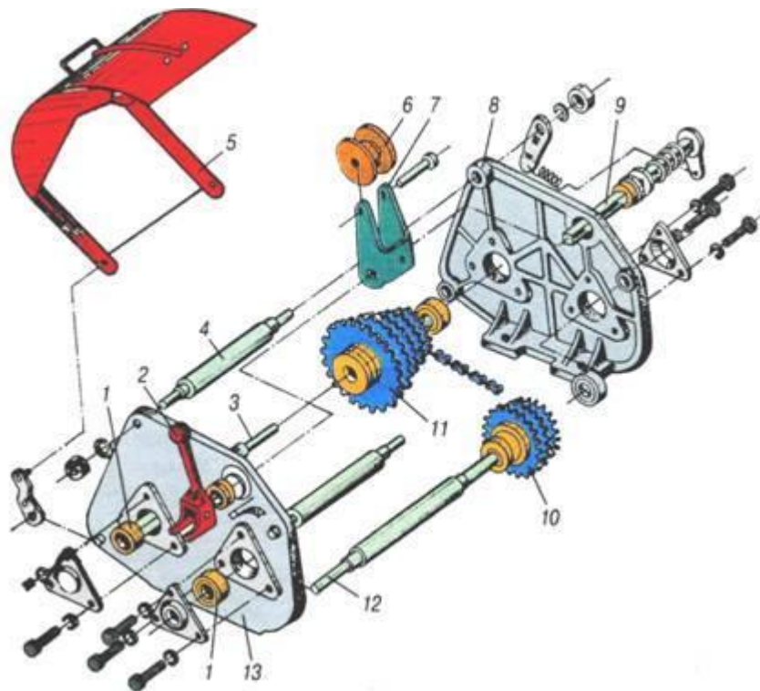
Рис. 4. Схема ланцюгового редуктора бурякових сівалок ССТ-12В і ССТ-8В:
