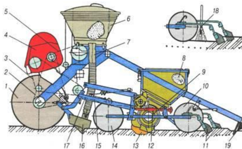
Рис. 3. Схема технологічного процесу роботи сівалок ССТ-12В і ССТ-8В
