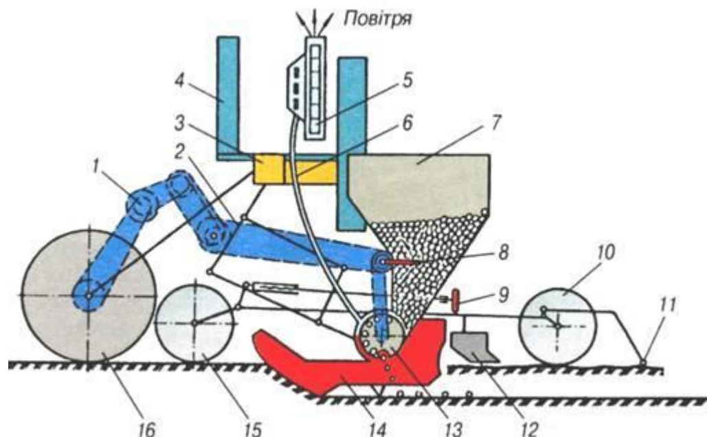
Рис. 9. Функціональна схема сівалки СУПО-6
