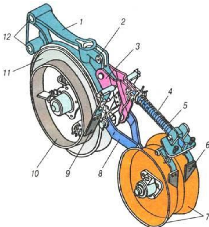
Рис. 8. Однорядковий дисковий сошник сівалки СОН-4,2
