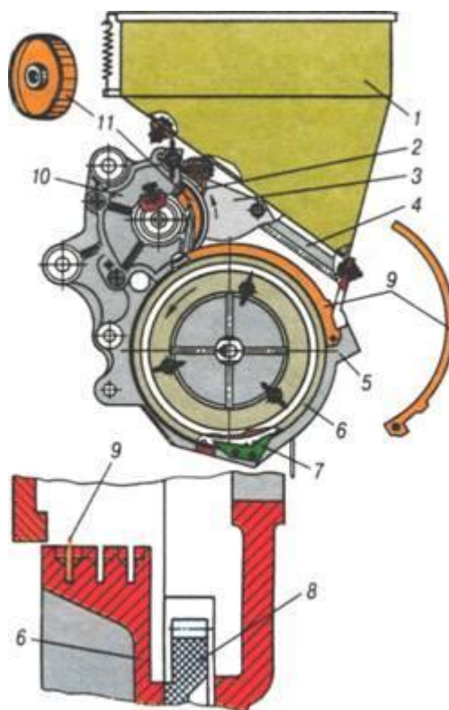
Рис. 15. Дисковий висівний апарат бурякових сівалок точного висівання ССТ-8В і ССТ-12В:
