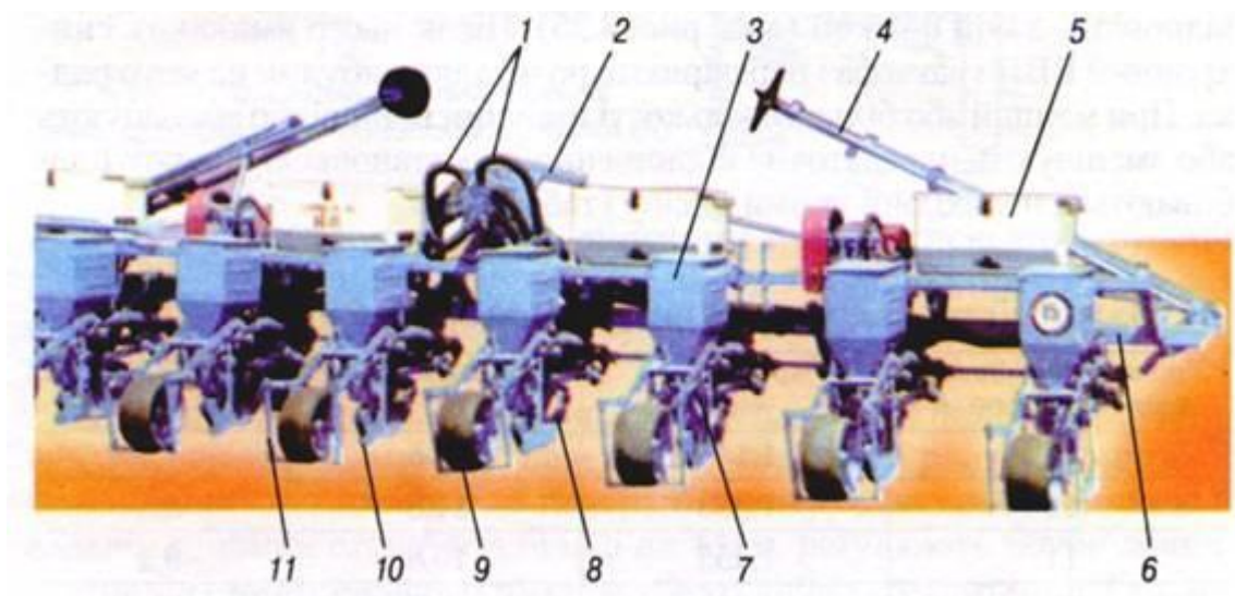
Рис. 1. Універсальна пневматична сівалка СУПН-8
