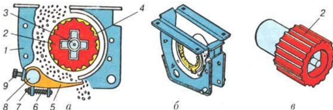
Рис. 17. Функціональна схема (а), коробка (б) і котушка (в) котушкового висівного апарата зі штампованою коробкою овочевої сівалки СОН-4,2
