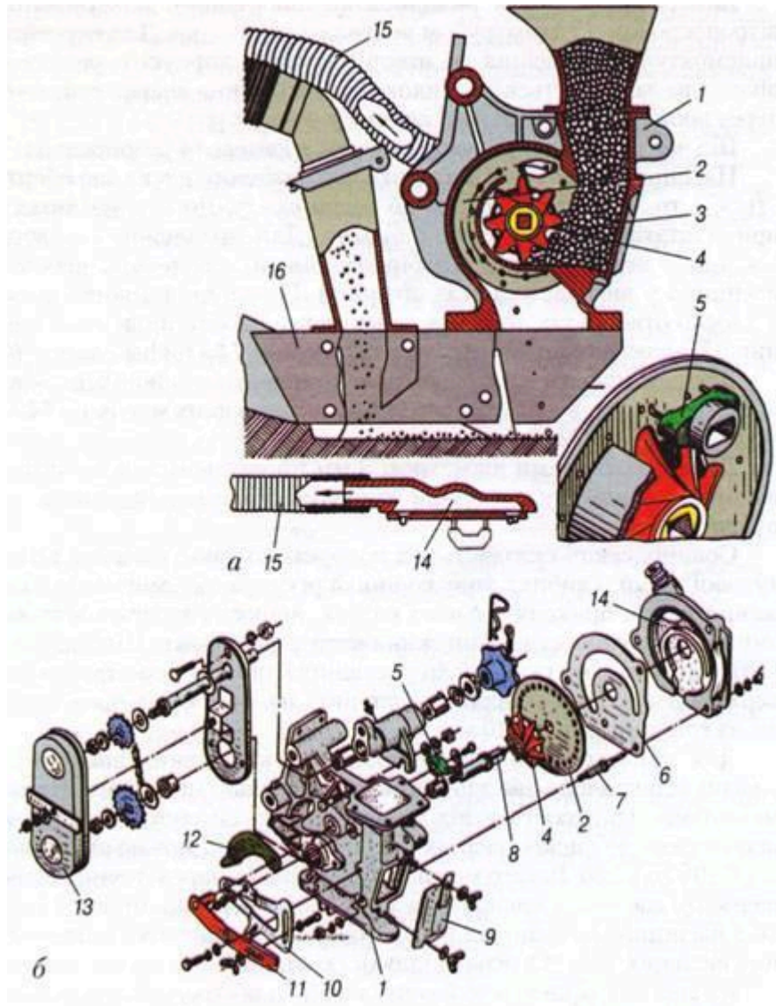
Рис. 13. Дисковий пневматичний висівний апарат сівалки СУПН-8А
