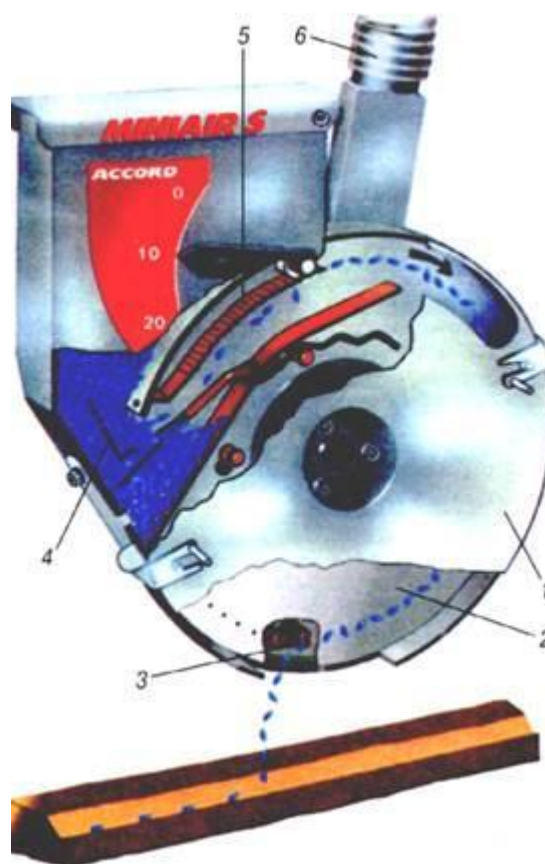
Рис. 18. Висівний апарат «MINIAIR S»:
