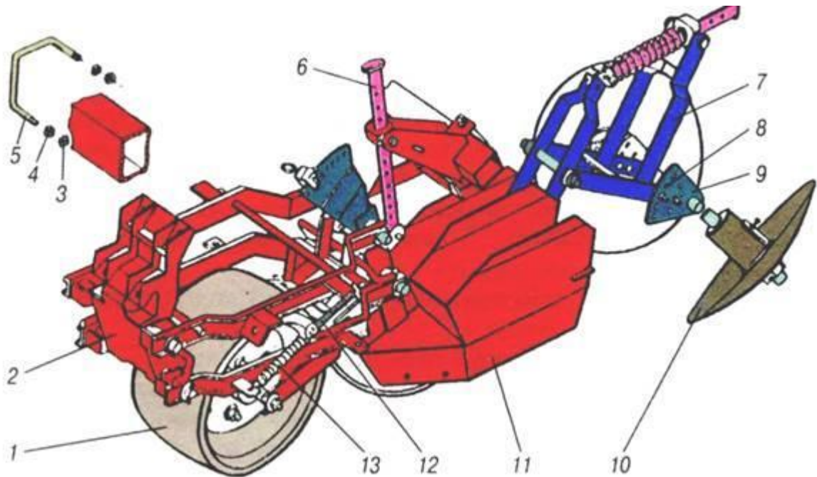
Рис. 11. Посівна секція сівалки СЛС-12
