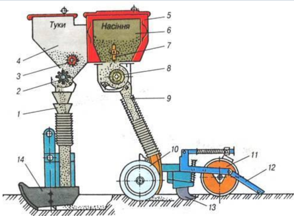
Рис. 6. Функціональна схема овочевочевої сівалки СОН-4,2
