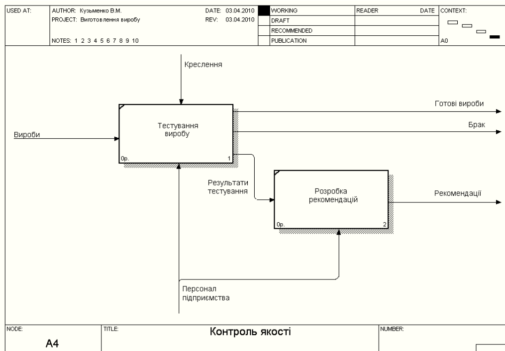
Рисунок 1.4 – Діаграма декомпозиції роботи «Контроль якості»
