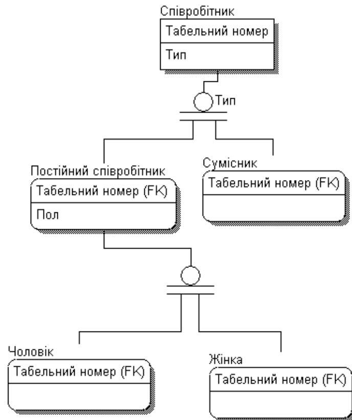
Рисунок 2.7 – Ієрархія спадкування. Комбінація повної та неповної категорій
