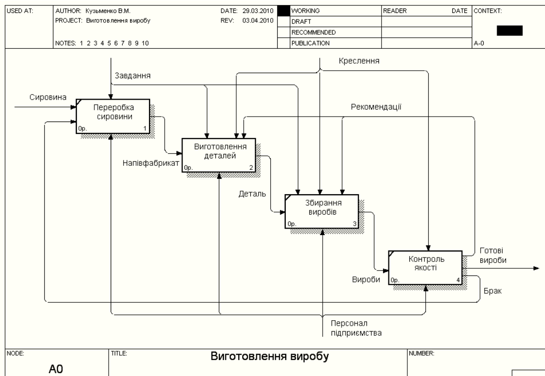
Рисунок 1.2 – Діаграма декомпозиції першого рівня
