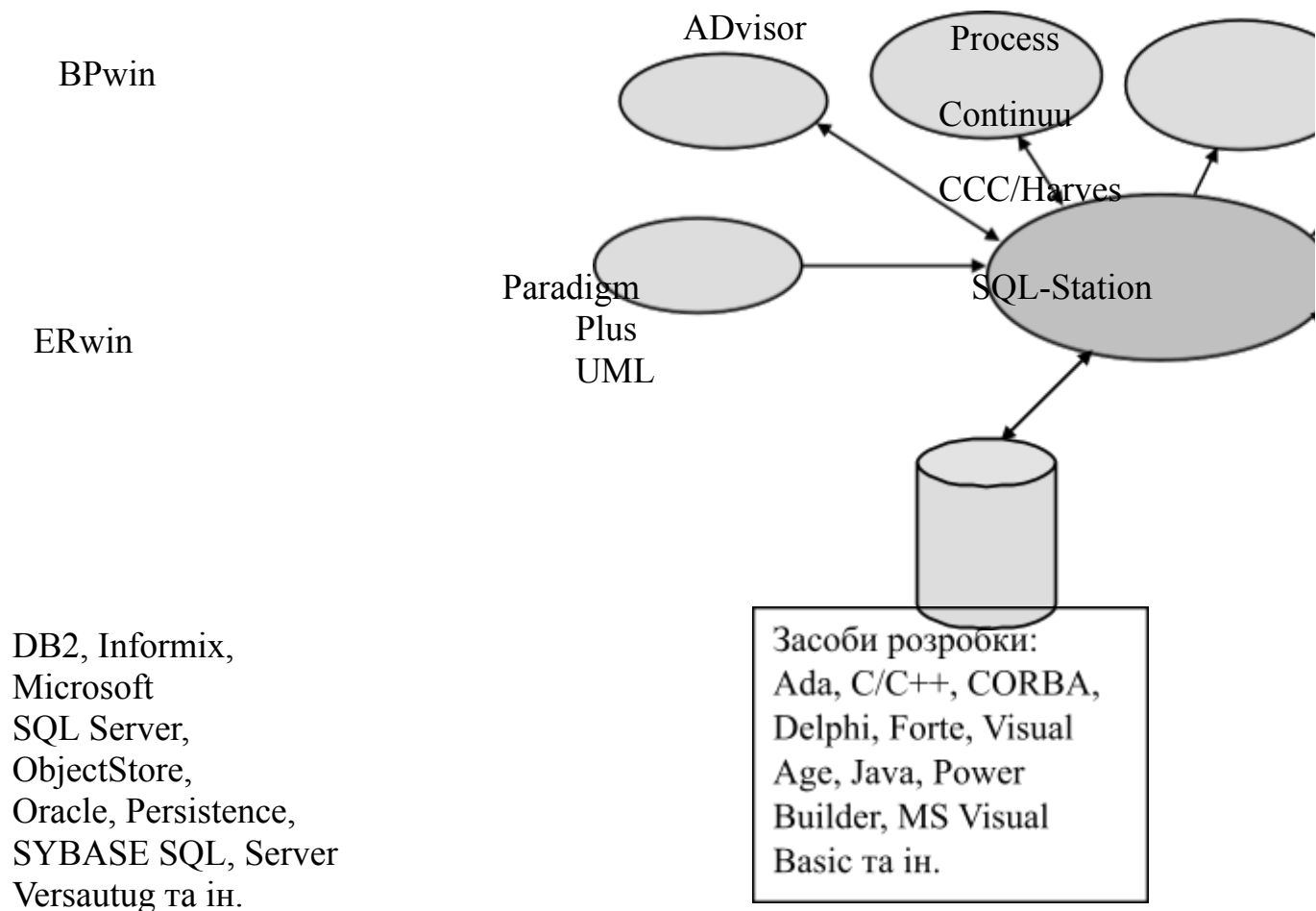
Рисунок 5.1 – Загальна схема взаємодії продуктів Computer Associates з Paradigm Plus
