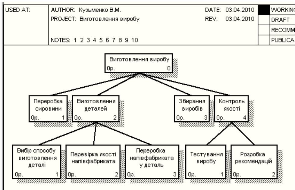
Рисунок 1.6 – Діаграма дерева вузлів (вид подання – за вибором)
