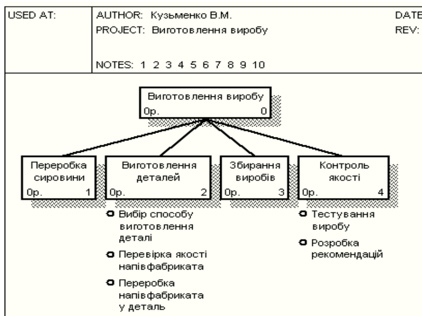
Рисунок 1.5 – Діаграма дерева вузлів (вид подання – за замовчуванням)
