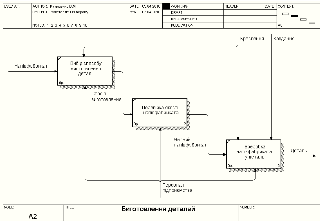
Рисунок 1.3 – Діаграма декомпозиції роботи «Виготовлення деталей»
