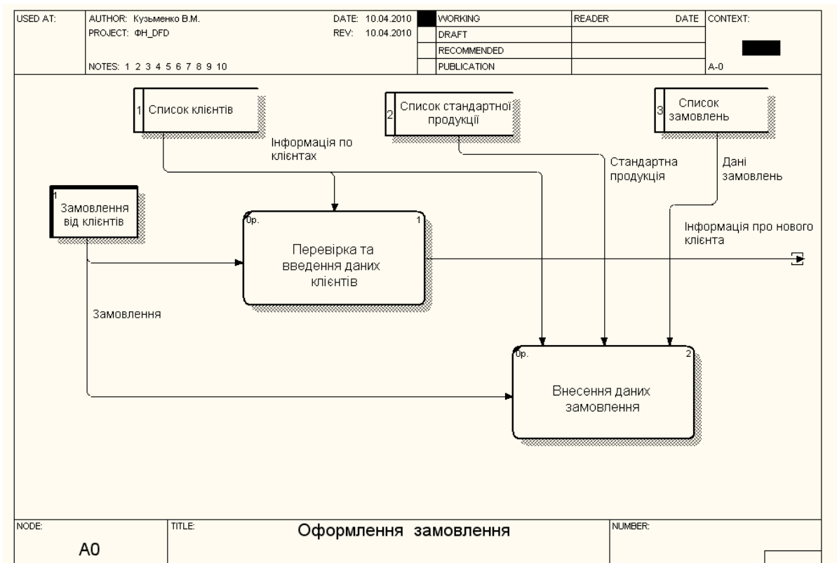
Рисунок 4.7 – Дочірня діаграма DFD для роботи «Оформлення замовлення»
