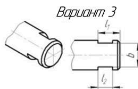
Варианты исполнения оси
