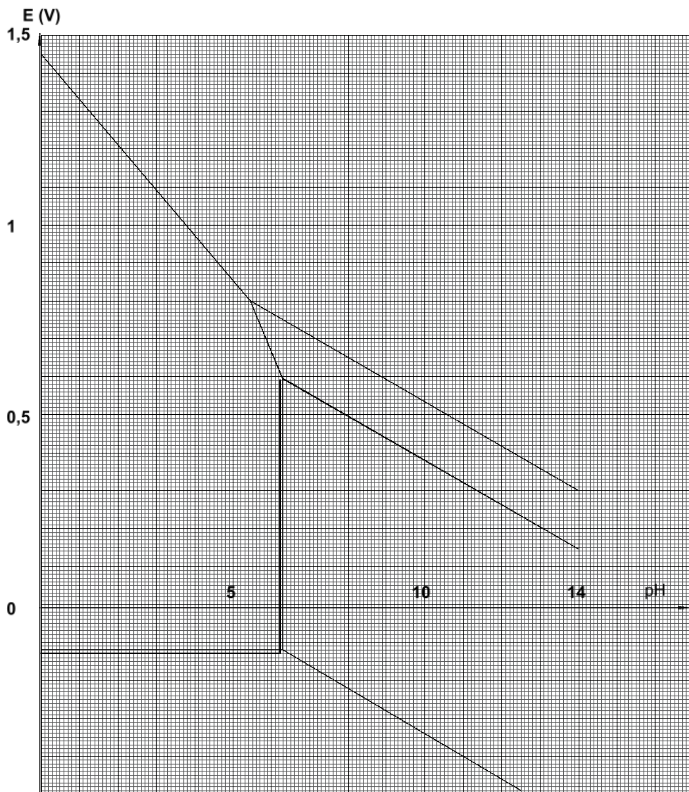
Figure 3 : Diagramme potentiel – pH simplifié de plomb
