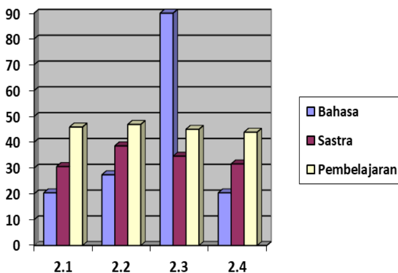
Gambar 1. Data Pembelajaran
