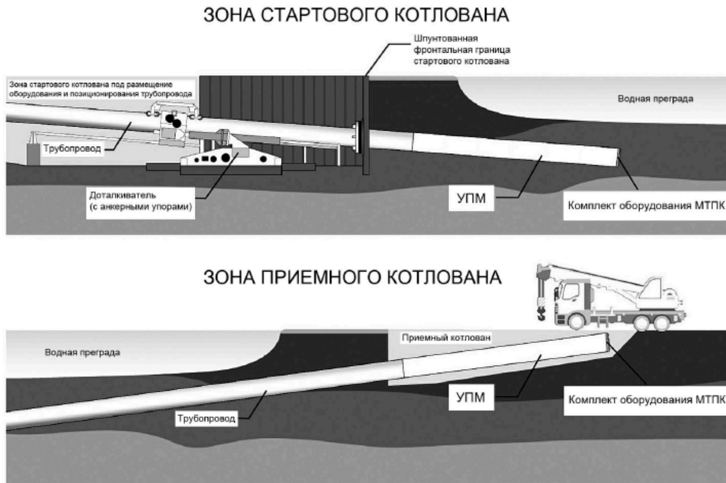
Рисунок 8.7 - Общая схема производства работ по технологии ГНБЦ
