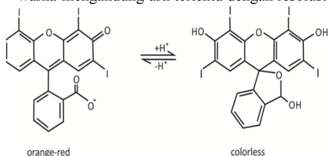
Gambar 1. Protonasi dan deprotonasi erythrosine
