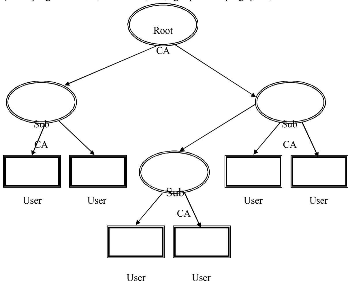
Hình 3-12: Mô hình của Root CA
