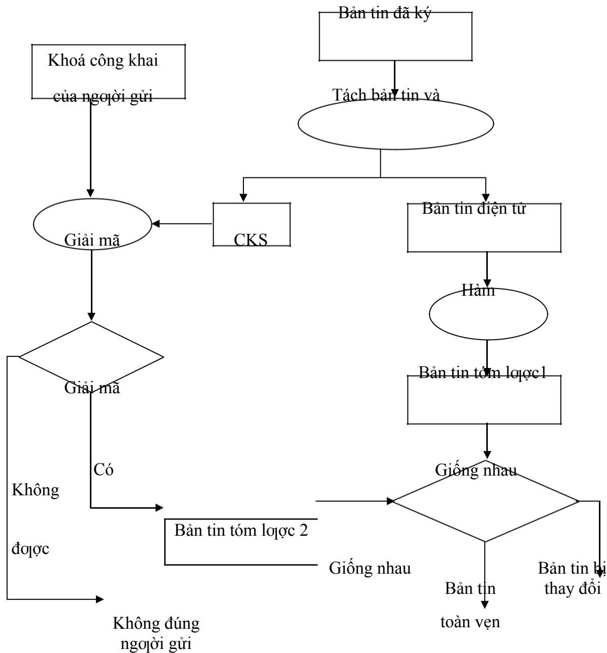
Hình 3-18: Quản lý khóa sử dụng Private Key
