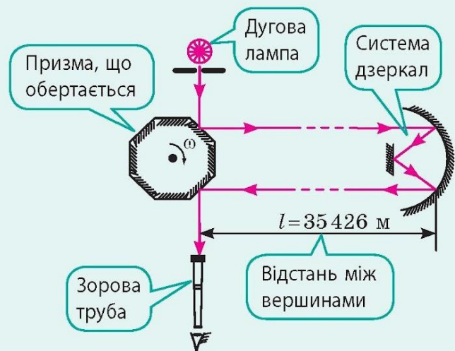
Схема дослідів А. Майкельсона
