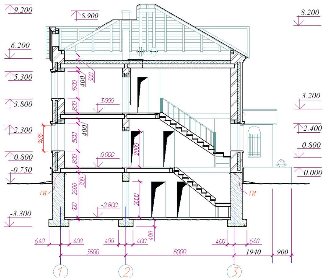
Рис. 4. Разрез 1-1 по лестнице в масштабе М 1:100
