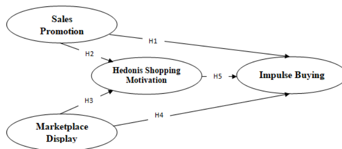
Gambar 1. Kerangka Konsep
