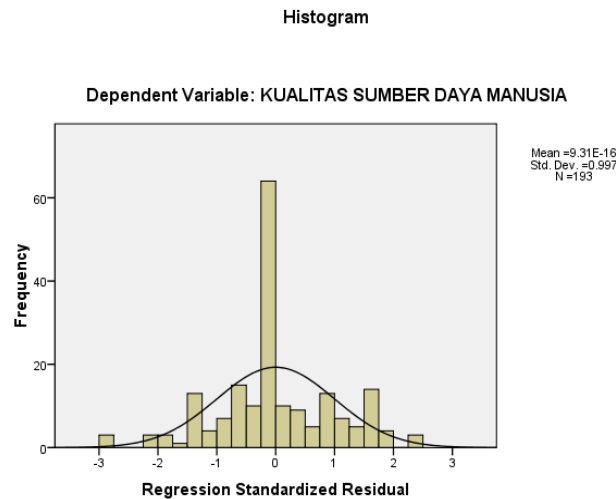
Gambar 1. Uji Normalitas
