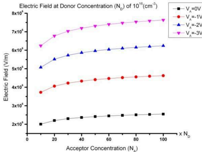
Gambar 1. Karakteristik konsentrasi-medan listrik
