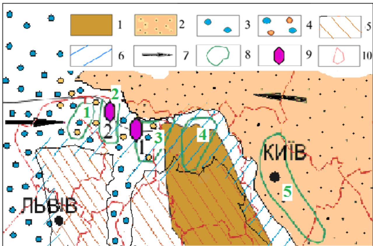
Рис. 5.3. Схема мірагенічного районування Прип'ятського бурштиноносного басейну (олігоцен) за [19]: 1 – Український щит; 2 – опріснені води епіконтинентального моря; 3 – солоні води Паратетису; 4 – область змішування солоних і опріснених вод; 5 – олігоценовий суходіл; 6 – ділянки періодичного затоплення суходолу; 7 – напрям течій; 8 – бурштиноносні зони: 1) Маневицько-Зарічнянська, 2) Володимирецько-Дубровицька, 3) Клесівсько-Пержанська, 4) Бараши-Лугинська, 5) Київсько-Дніпровська; 9 – родовища бурштину: 1) Клесівське, 2) Вільне та Володимирець Східний; 10 – межі адміністративних областей України
