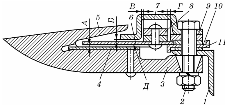
Рис. 8.4. Різальний апарат :
