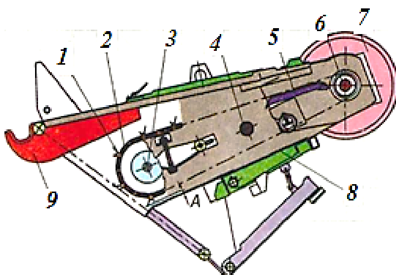
Рис. 8.6. Похила камера: 1 — планка (гребінка); 2 — ланцюг транспортера; 3 — нижній ведений вал; 4 — контрпривідний вал; 5 — напрямна; 6 — верхній ведучий вал; 7 — шків; 8 — корпус; 9 — опора захвату
