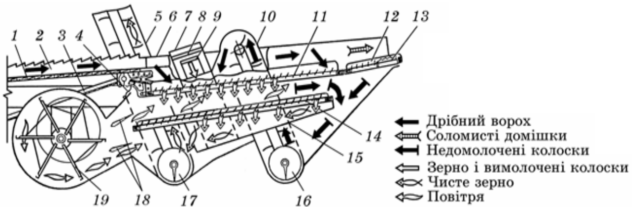
Рис. 8.11. Схема роботи очисника комбайна КЗС -9-1:
