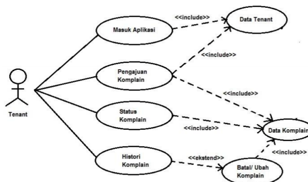
Gambar 1. Use Case Diagram (Sumber: Nama Penulis, Tahun)
