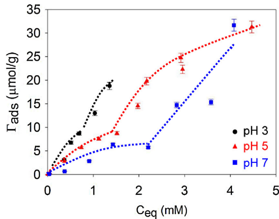
Figura 1. Isothermas de adsorción
